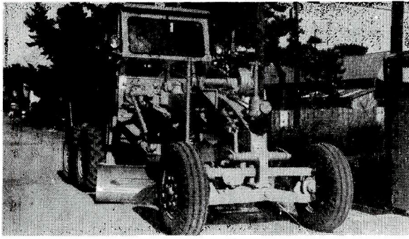
このほど市役所建設課ではモータグレーダを400万円で購入、道路や悪路の補修に大きな威力を発揮しております。 この機械の用途はたいへん広く、路面切削作業、斜面切削、溝堀作業、現場混合作業等に使われます。
