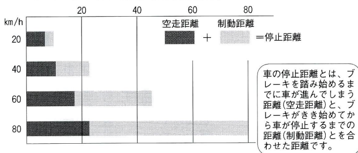
〔2〕車の停止距離（高萩警察署資料）
