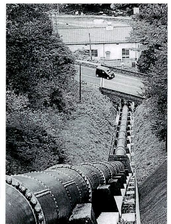
水圧鉄管 直径約1mの鉄管が約77mの落差を下ります。
