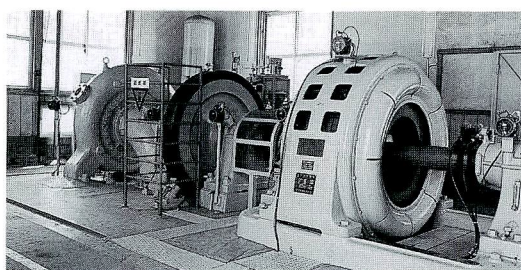
水車と発電機 左奥のかたつむりの形をしているのが水車で、同軸で回る右端が発電機。
