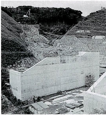
えん堤の基礎工事が進む工事現場
