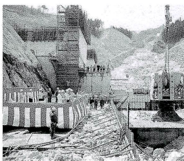
②コンクリート打設開始
