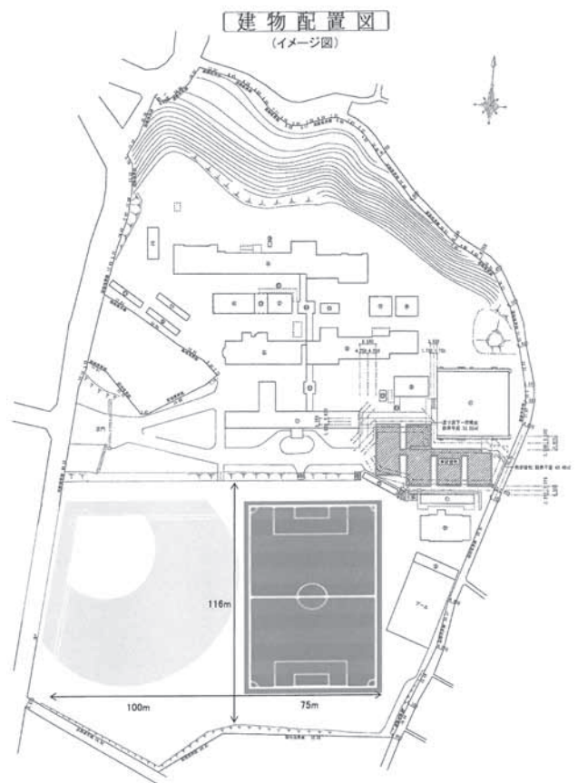
人工芝グラウンドのイメージ図
